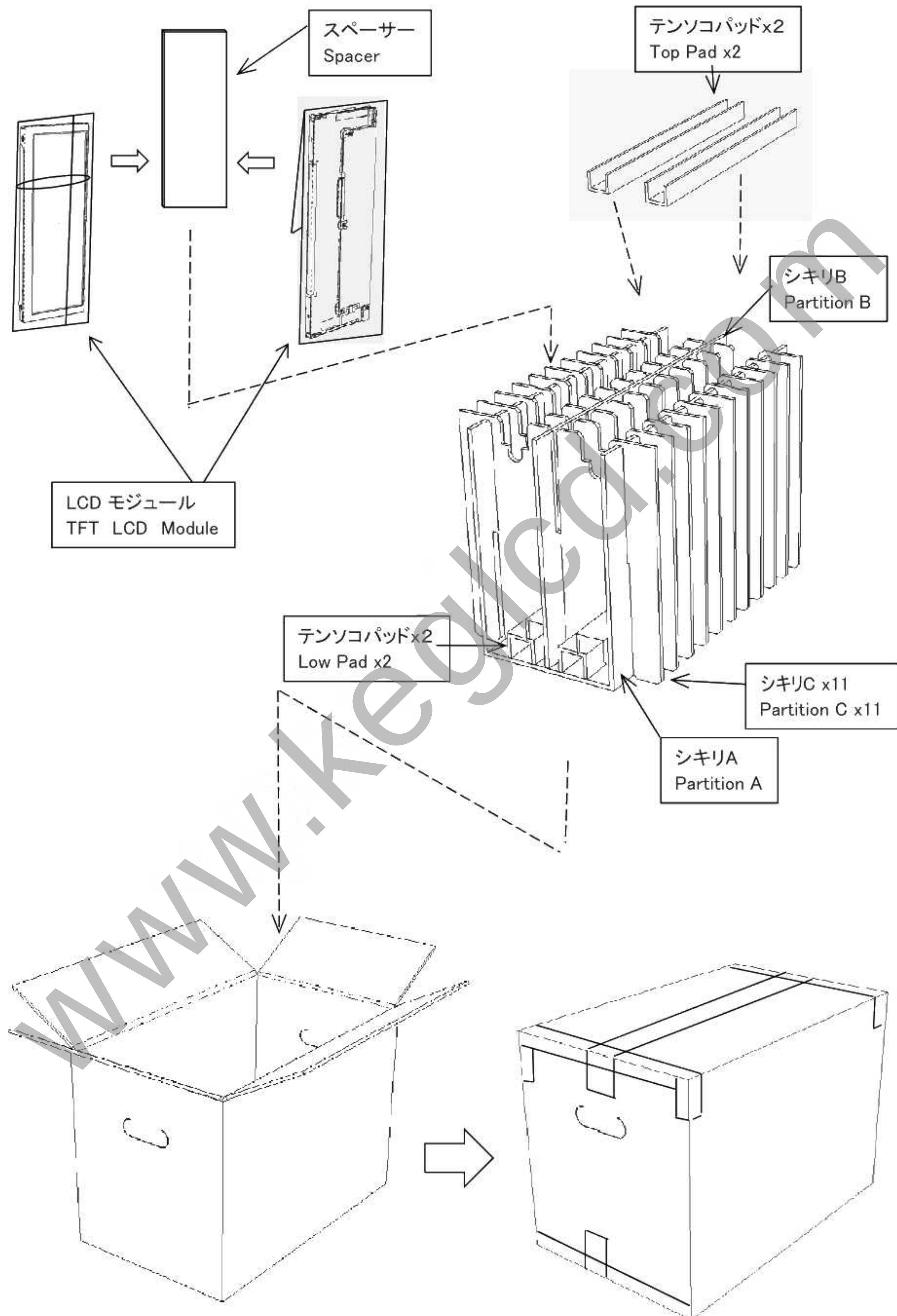
図3: 包装組品図 (Fig3. Packing Form)
